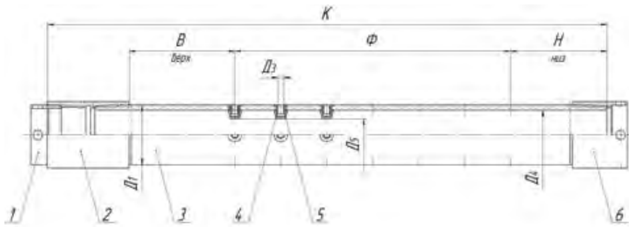
1. Заглушка 2. Муфта 3. Корпус 4. Полая пробка 5. Втулка 6. Заглушка
