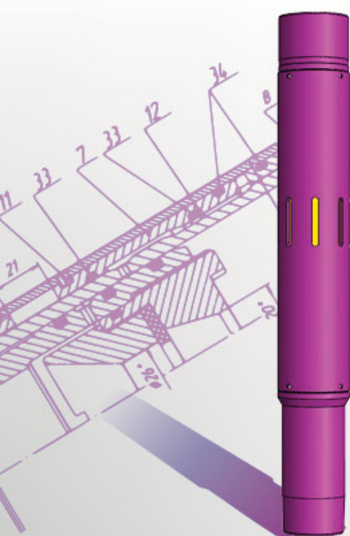
Муфта ступенчатого гидроразрыва пласта управляемая МСГРП-У
